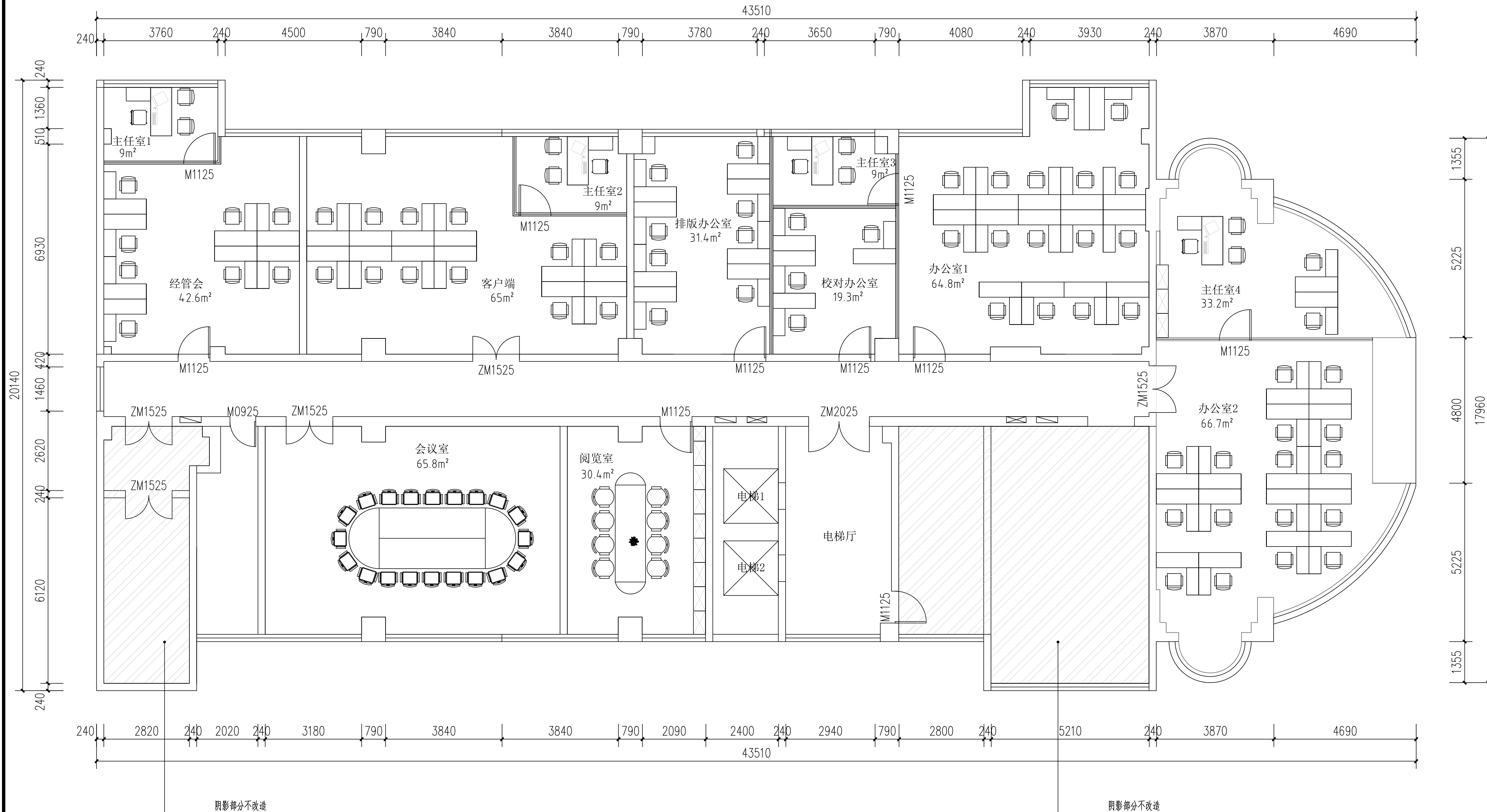
五层平面布置图 1:100
